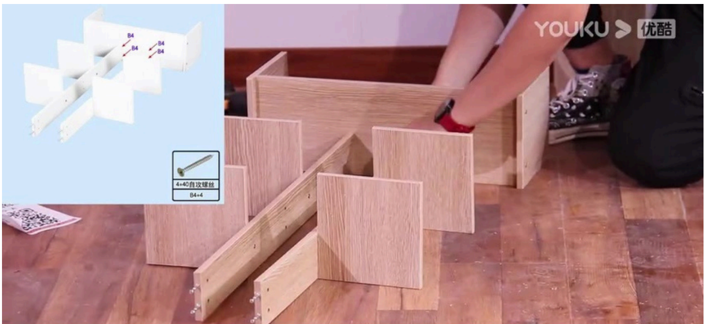
Pasul 12: Prinde materialul textil (dacă există) pe cadru.
